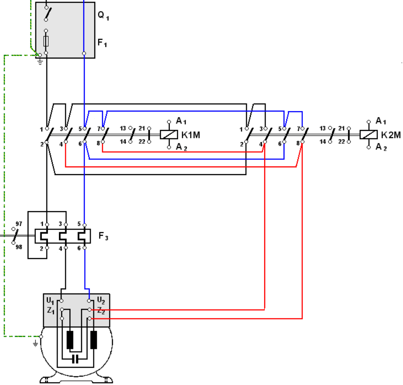
ΣΧΕΔΙΟ 8 ΑΛΛΑΓΗ ΦΟΡΑΣ ΠΕΡΙΣΤΡΟΦΗΣ ΜΟΝΟΦΑΣΙΚΟΥ ΑΚΒΔ ΚΥΚΛΩΜΑ ΚΥΡΙΟ
